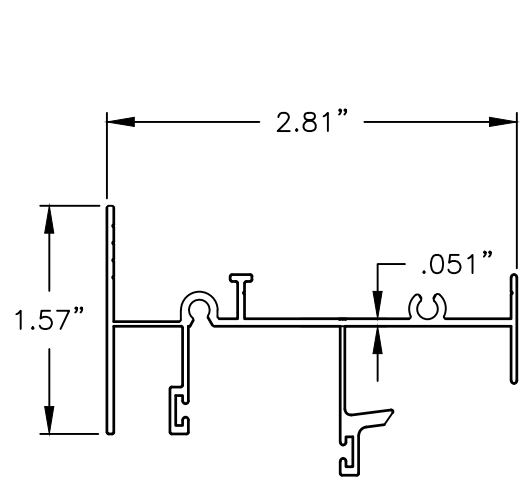
HEAD 6063-T5
