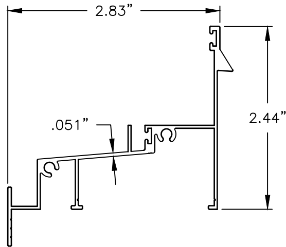
SILL 6063-T5
